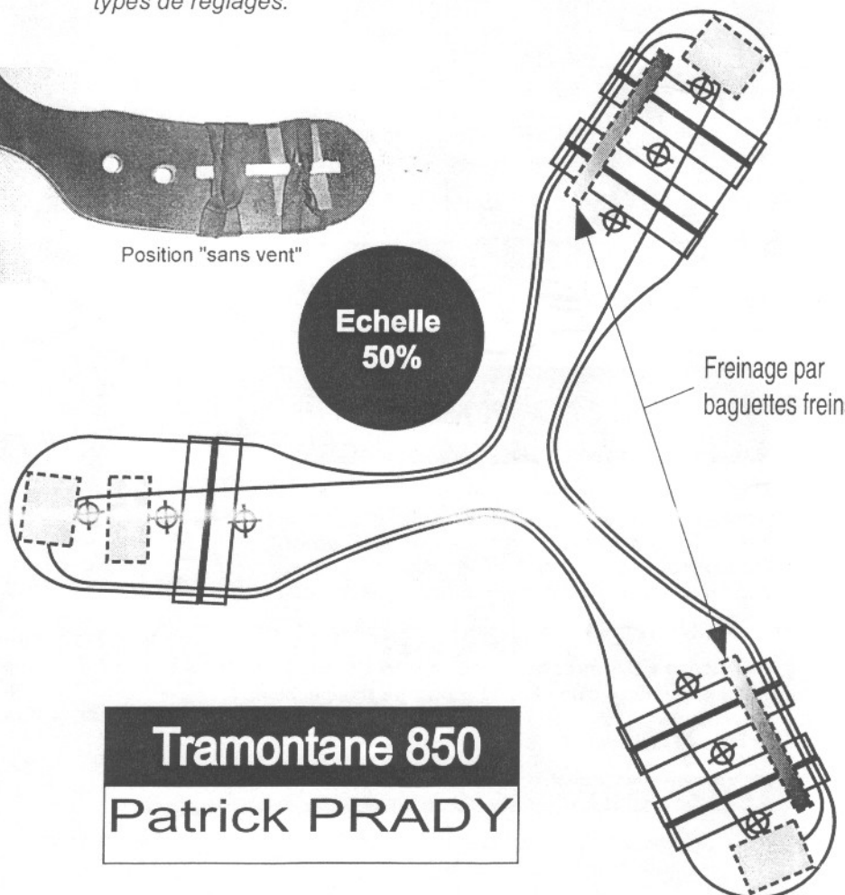
Vues de l'intrados avec les deux types de réglages.
